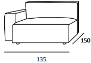
CHAISE LONGUE MAX 1 L/R ARM
